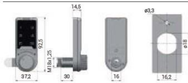
SOFT CE1034 Διαστάσεις (σε mm)
