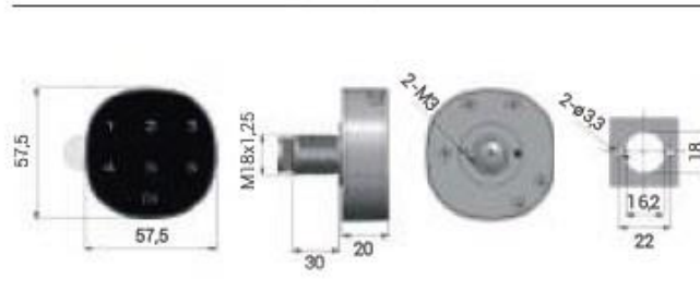
PUCK CE2032+U Διαστάσεις (σε mm)
